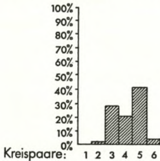
Abb. 14. Die Prozentanteile von Kreispaaren an Zwiebelknopffibeln des Typs 3, Var. B.
