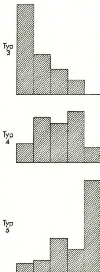
Abb. 22. Zeichnerische Darstellung der in Abb. 21 errechneten relativierten Anteilwerte.
