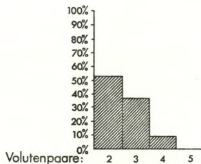
Abb. 16. Die Prozentanteile von Volutenpaaren an Zwiebelknopffibeln des Typs 4, Var. B.
