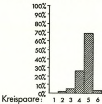
Abb. 15. Die Prozentanteile von Kreispaaren an Zwiebelknopffibeln des Typs 4, Var. A.
