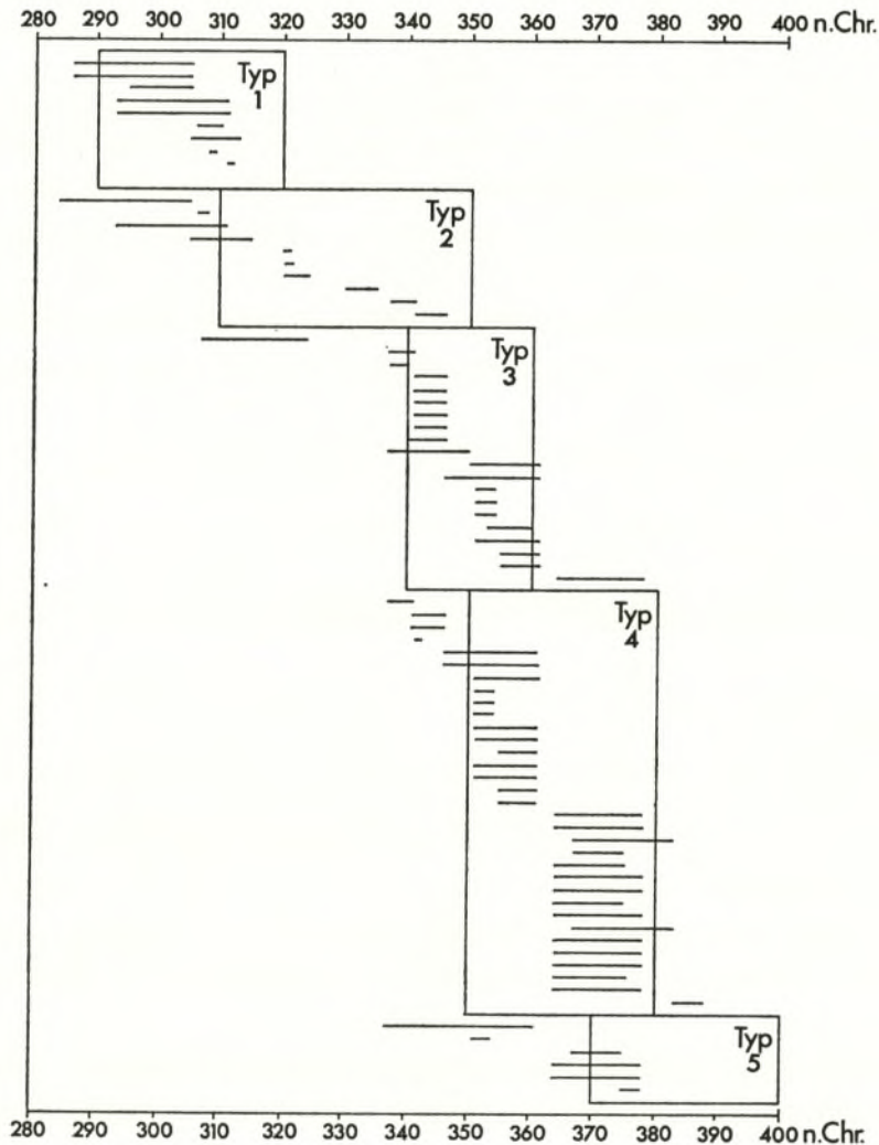
Abb. 12. Die Prägezeiten der mit Zwiebelknopffibeln vom Typ 1 bis 5 kombinierten Schlußmünzen. Die eingegrenzten Felder bezeichnen die als Datierung verwendeten Zeitspannen.
