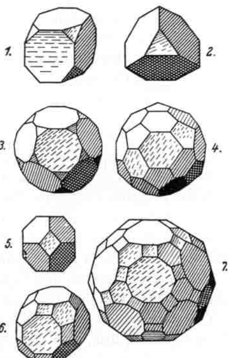
XI. Rhombicosidodecaedron.
