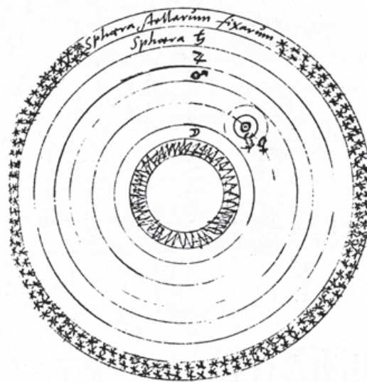
Abb. 109: Rothmann, Astronomia fol. 16r. Rothmanns früherer Versuch eines geoheliozentrischen Weltbildes (nach Martianus Capella), beschränkt auf die unteren Planeten Merkur und Venus, die um die Sonne kreisen; die 3 äußeren Planeten kreisen noch um die im Zentrum stehende Erde. Landes- und Murhardsche Bibliothek Kassel, 4° Ms. astron. 11. Aus Schofield 1981, plate 2. Siehe auch Granada/Mosley/Jardine 2014, S. 15.
