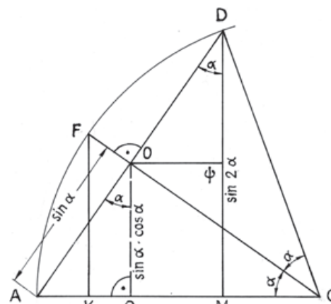
Abb. 74: Halbwinkelformel.
