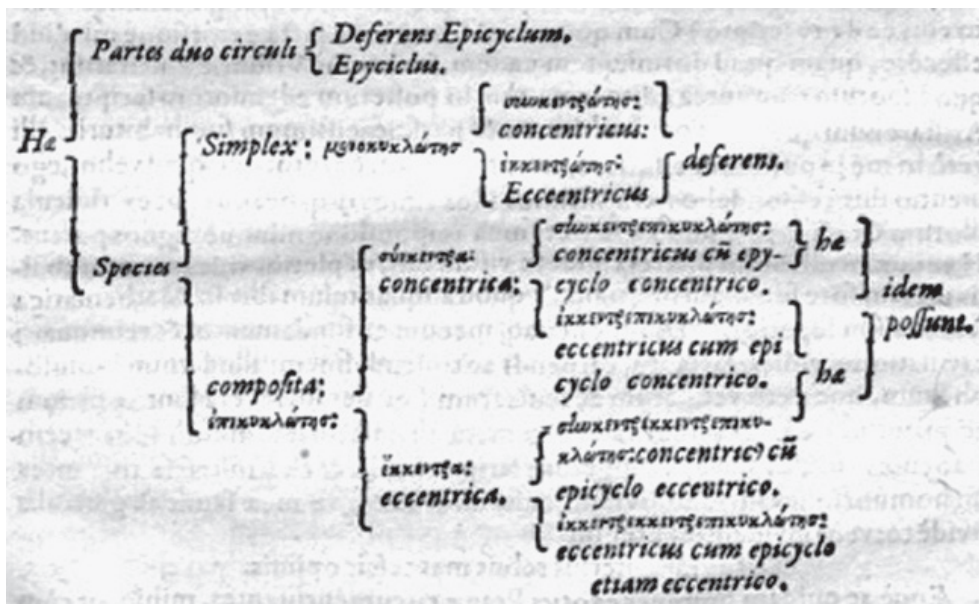
Abb. 55: Formen astronomischer Hypothesen, Blatt H2r.
