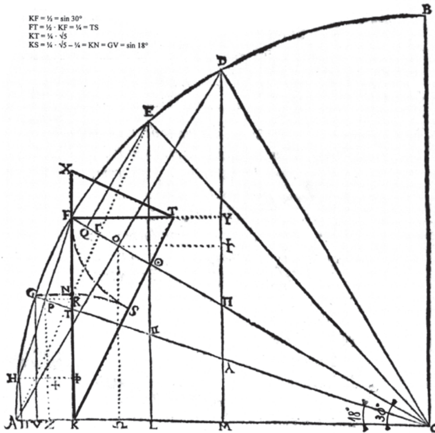
Abb. 83: Diagramm K4r. Ich habe darin die Konstruktion von \sin 18^\circ hervorgehoben. \sin 18^\circ = GV = KN = KS = KT - TS = KT - TF = \frac{1}{4} \cdot (\sqrt{5} - 1) . Der Schnittpunkt von PZ und HΦ ist Ψ, das Symbol + ist ein Druckfehler. Der Punkt unterhalb von H auf AC heißt U.
