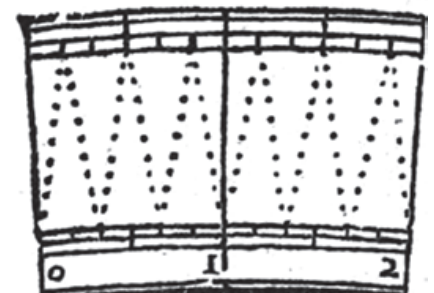
Abb. 39: Transversalteilung nach Rothmann. Ableseung 3° 27'. Aus Hamel 1998, S. 20.
