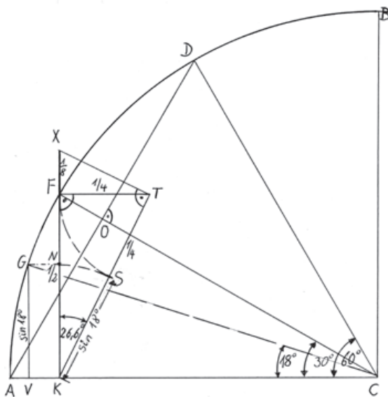
Abb. 72: Konstruktion der Seite des regelmäßigen Zehnecks, mit Dreieck KTF aus Diagramm K4r.
