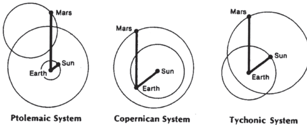
Abb. 25: Die Sichtwinkel von der Erde zu Sonne und Mars sind in allen drei Systemen gleich. Aus Gingerich 1992, S. 252.
