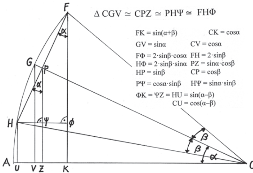
Abb. 78: Mittelwert. Blatt K4r Ausschnitt.
