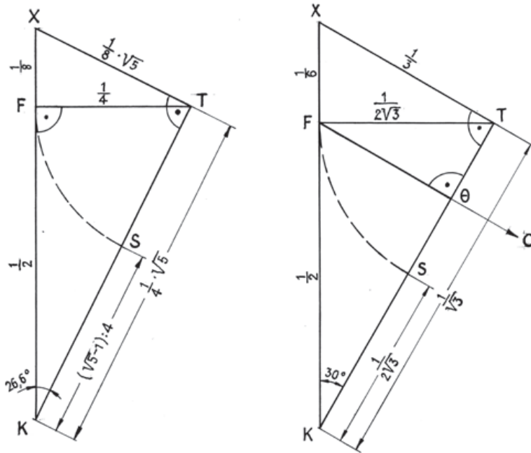
Abb. 81: Auszug aus Diagramm K4r. Dreieck KTX für \sin 18^\circ .
