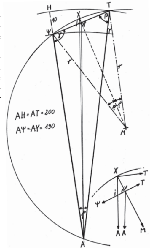
Abb. 42: Zur Berechnung des Ablesefehlers bei geradliniger Transversalteilung nach Ursus, Fundamentum Astronomicum , Blatt Glr.
