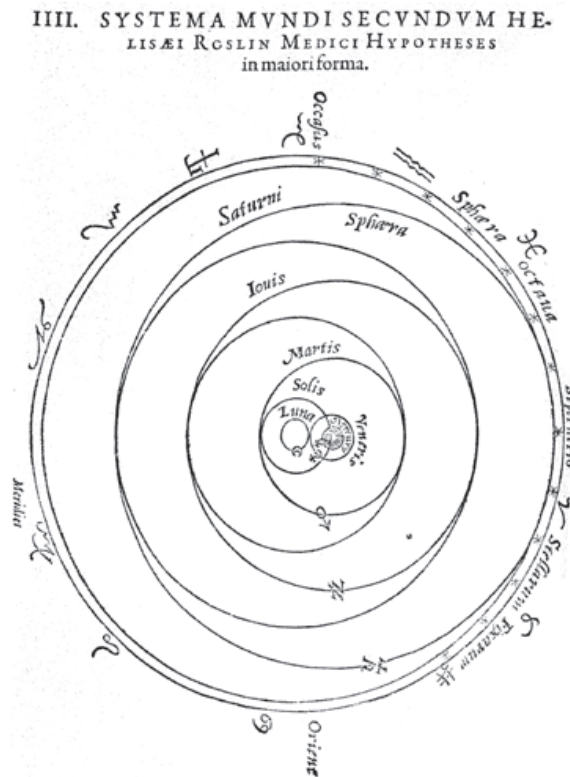
Abb. 52: Weltsystem von Röslin, De Opere Dei 1597, S. 56.
