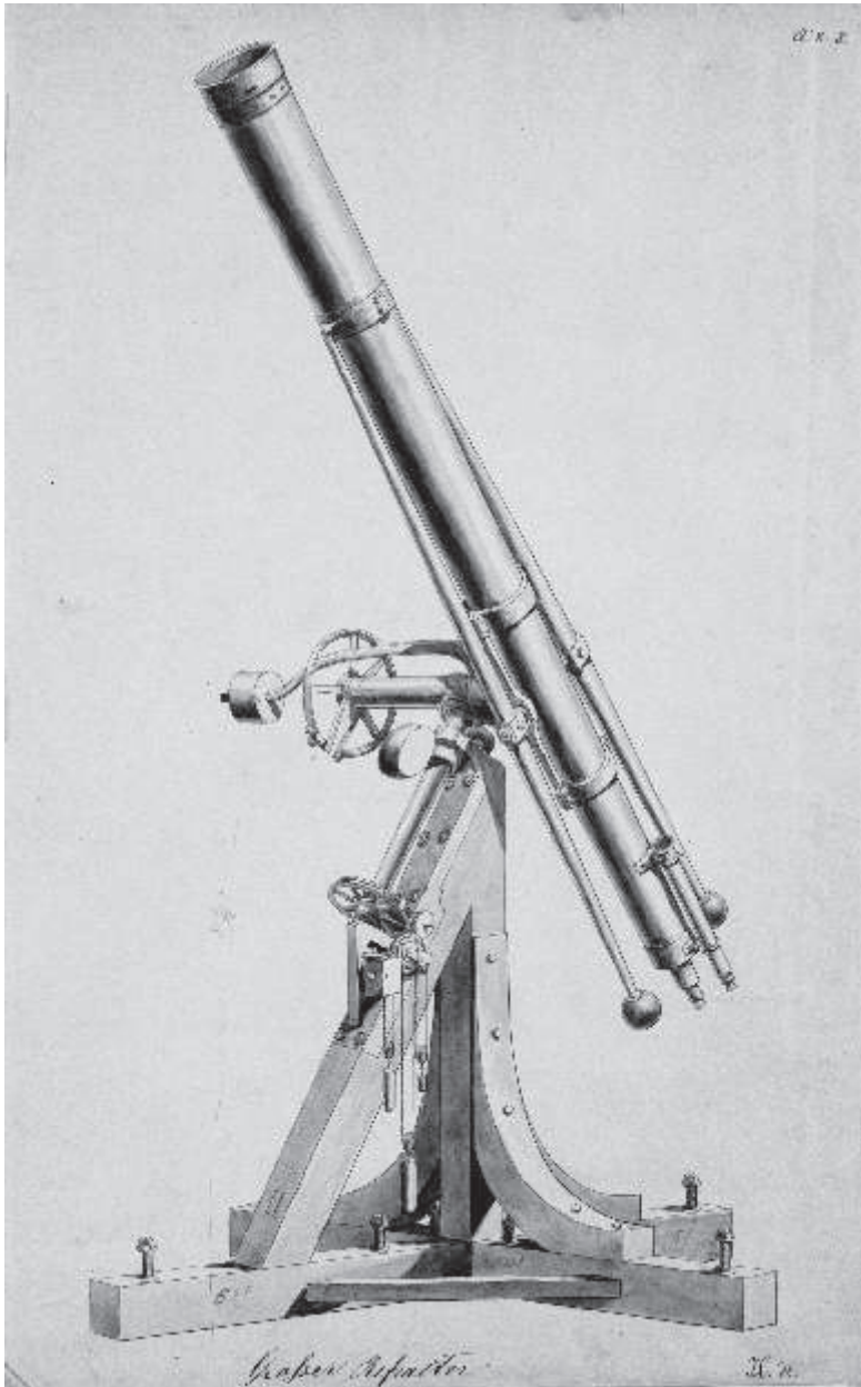
Die von Liebherr erstellte Lithografie stellt sowohl den 1824 fertig gestellten Dorpater Refraktor als auch den weitgehend baugleichen Refraktor für Berlin (1829) dar; mit Letzterem gelang Galle 1846 die Entdeckung des Planeten Neptun.
