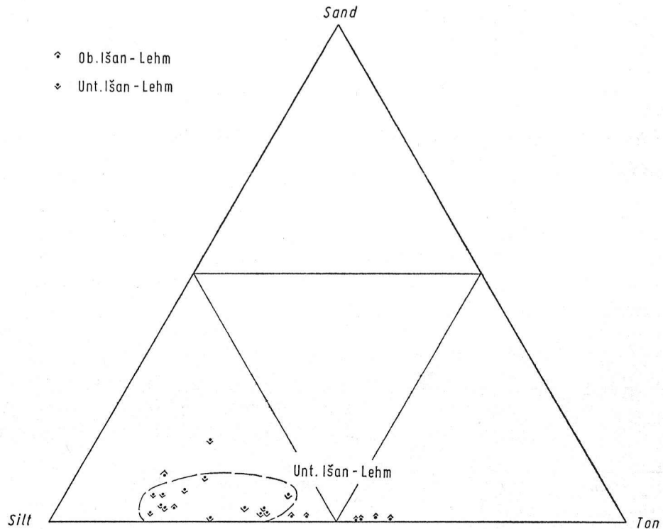
Abbildung 34. Kornverteilungsdiagramm der gleybegleitenden Lehme der İsan-Schichten der Kanalprofile km 37,13, 38,51, und 40,0 bei İsan Bağıryāt.
