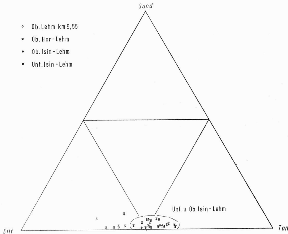
Abbildung 33. Kornverteilungsdiagramm der gleybegleitenden Lehme der Kanalprofile km 9,55, 37,13, 38,51 und 40,0 bei Işān Baḥrīyāt.
