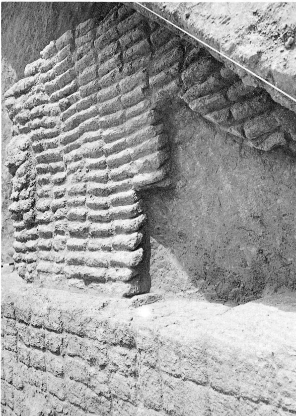
1 Ziegelstapelung für Ausbesserung an der Temenos-Mauer
