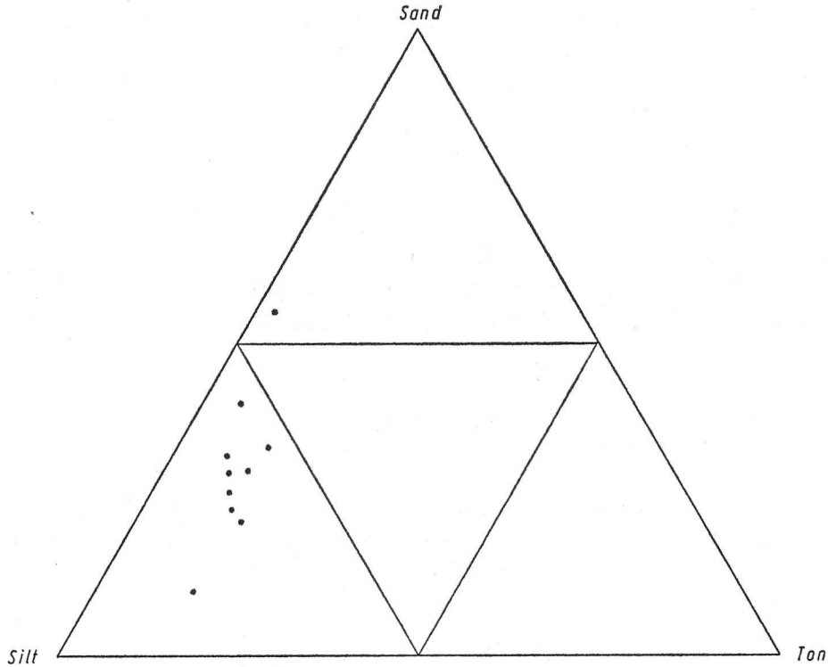
Abbildung 37. Kornverteilungsdiagramm der nach-Isin-zeitlichen Tellversturz- und Tellverspülsedimente im Profil Isin 1 im Nordbereich des Tells.
