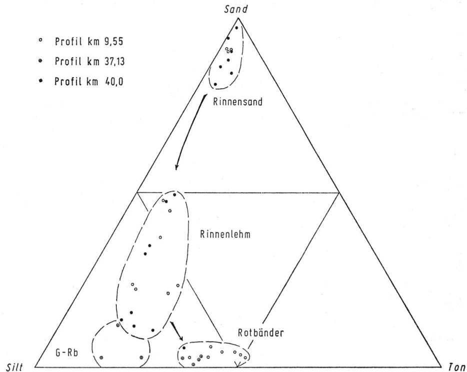
Abbildung 31. Kornverteilungsdiagramm der Rinnensande, Rinnenlehme und Rotbänder-Schichten der Kanalprofile bei Išān Bahriyāt. G-Rb = Gelber Lehm der Rotbänder-Schicht im Profil km 37,13.
