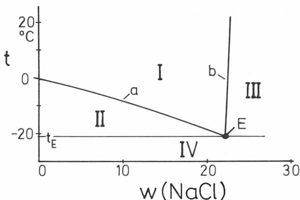
Bild 7: Schmelzdiagramm von Eis und Kochsalz. a) Schmelzpunktniedrigung; – b) Löslichkeit von NaCl in Wasser, E eutektischer Punkt mit der Temperatur t_E , w(\text{NaCl}) in g anhydr. Substanz in 100 g Lösung.
