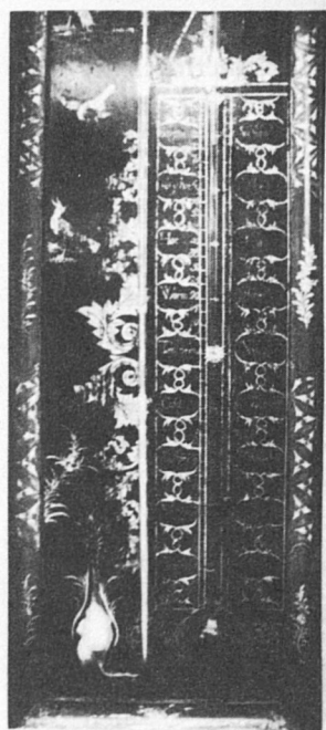
Bild 6: Weingeistthermometer von 1719 mit „Florentiner Skala“. Links unten Syphon eines Barometers. Science Museum, London.
