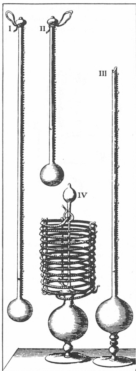
Bild 3: Florentiner Thermometer. I 100 Grad; – II 50 Grad; – III 300–400 Grad; – IV Spiralthermometer [Photo Istituto e Museo di Storia della Scienza di Firenze].
