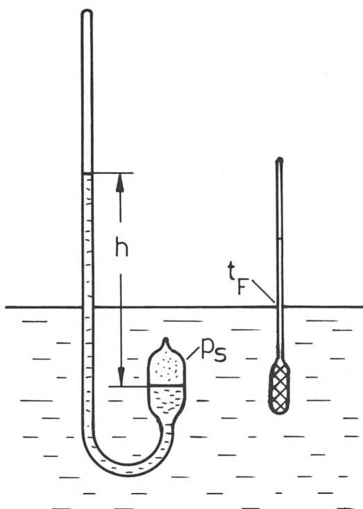
Bild 10: Apparatur zur Messung des Dampfdrucks von Wasser, 1723. Das linke Glasrohr ist 130 cm lang. Nicht maßstäblich. h Höhe der Quecksilbersäule, p_s Sättigungsdruck des Wassers, t_F Fahrenheittemperatur.
