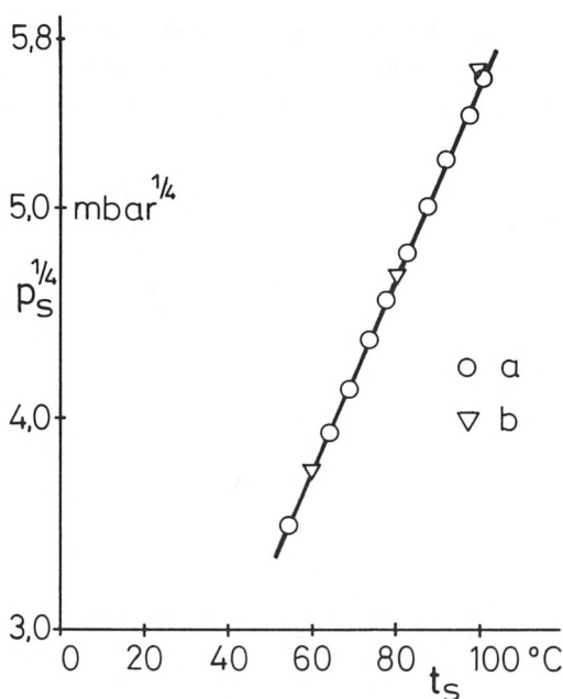
Bild 13: p_s^{1/4} als Funktion der Sättigungstemperatur t_s nach Fahrenheit. Kreise Fahrenheit's Werte, Dreiecke heutige Werte.
