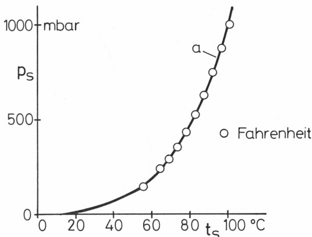
Bild 12: Fahrenheit's Dampfdruckwerte (Kreise) und heutige Dampfdruckkurve (ausgezogene Linie) im p, t -Diagramm.
