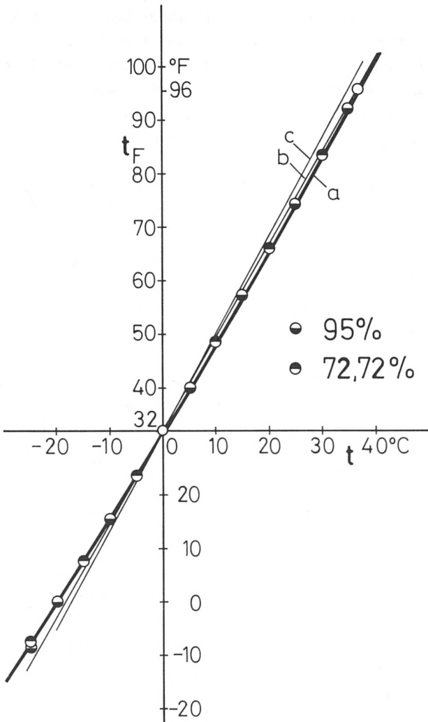
Bild 8: Skala der korrespondierenden Thermometer (Halle 1714) für Weingeist von 95% und 75,72% als Funktion der Celsius-temperatur.
