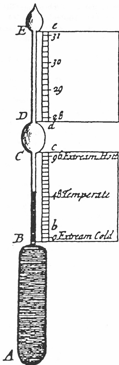
Bild 14: Hypsobarometer nach Fahrenheit, 1724.
